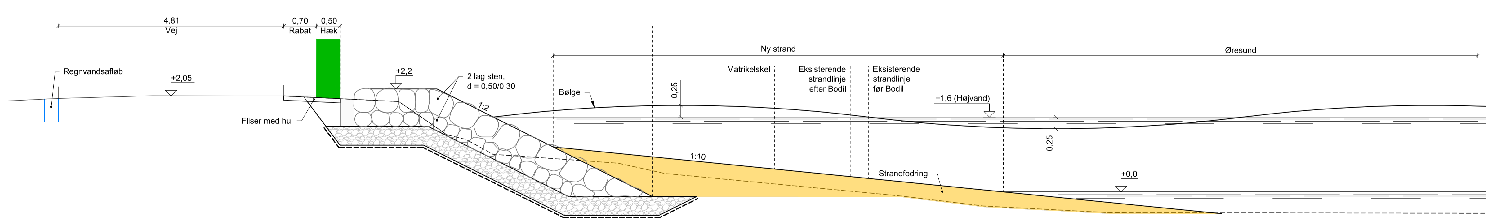
TVÆRSNIT A-A, 1:50
